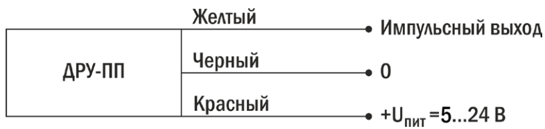
Рис. 3 – Схема подключения
